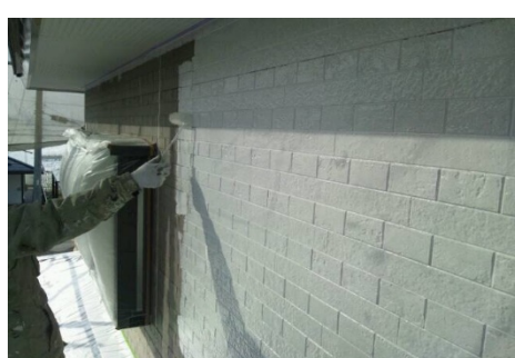
外壁：下塗りシーラー施工中
