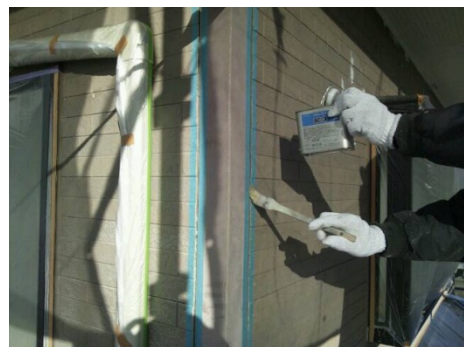
目地：接着プライマー塗布
