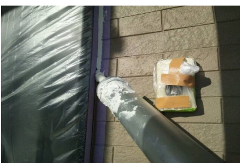
サッシ廻り：増し打充填
