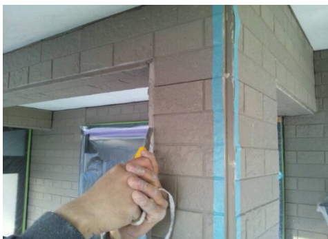
目地：破断部Vカット
